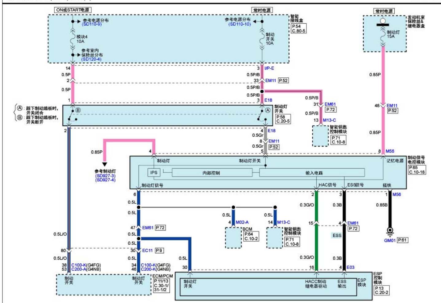
电控稳定程序(ESP)系统(2)
